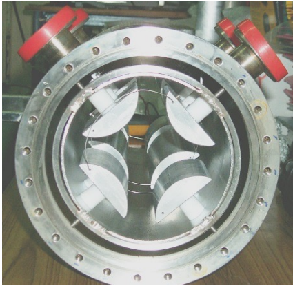
quadrupole
